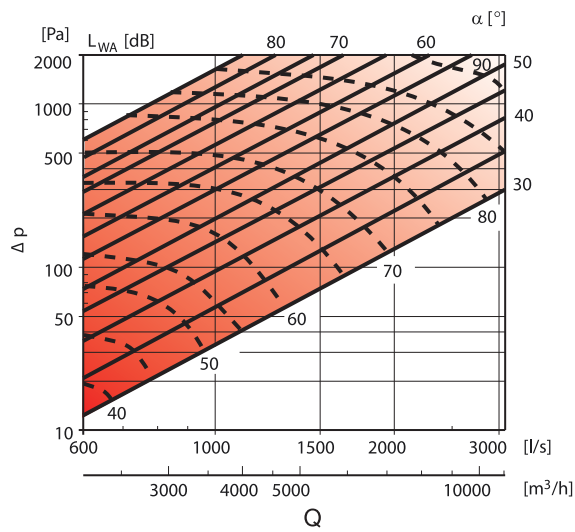
AKH Ø500
