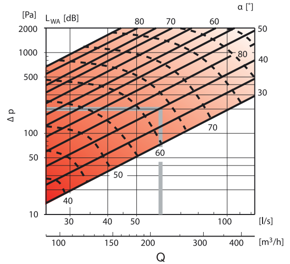
AKH Ø160
