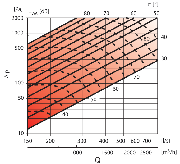
AKH Ø250
